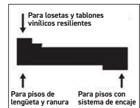
Diseño de borde combinado
